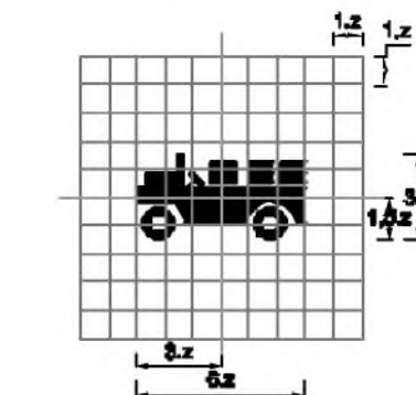
Biển số P.140: Cấm xe công nông và các loại xe tương tự
