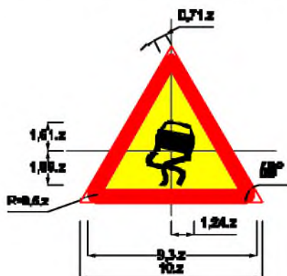
Biển số W.222a: Đường trơn
