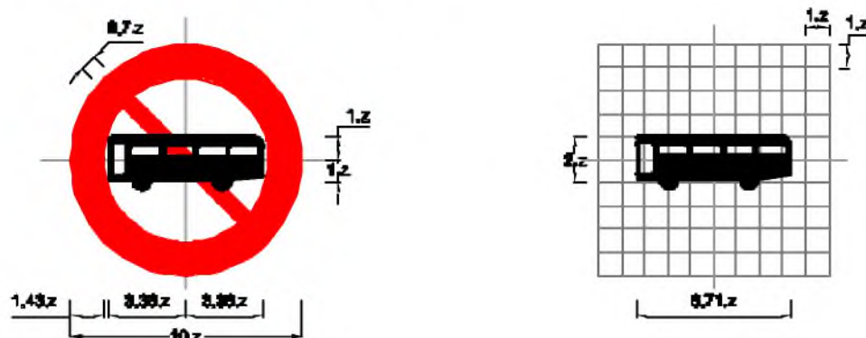
Biển số P.107a: Cấm xe ô tô khách
