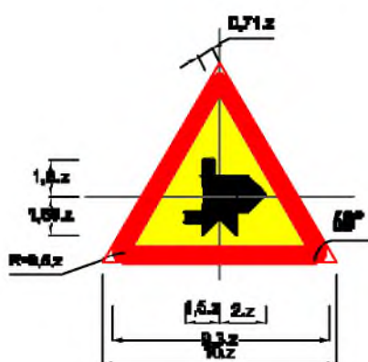
Biển số W.207: Giao nhau với đường không ưu tiên
