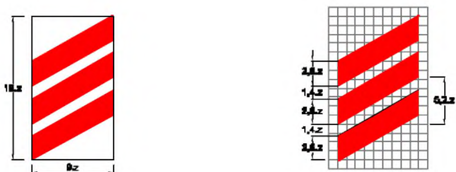
Biên số W.243c: Nơi đường sắt giao không vuông góc với đường bộ
