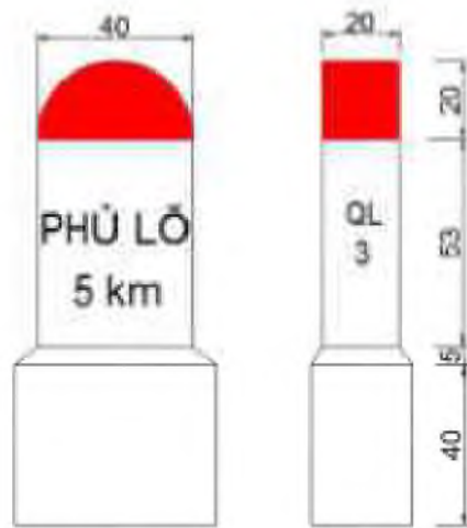
Ghi chú: Kích thước ghi trên hình vẽ là cm Hình I.1 - Cột kilômét dạng cột thấp
