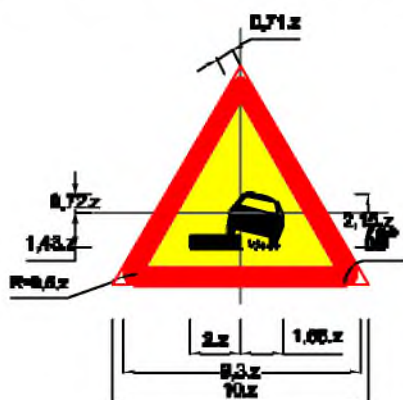
Biển số W.222b: Lề đường nguy hiểm
