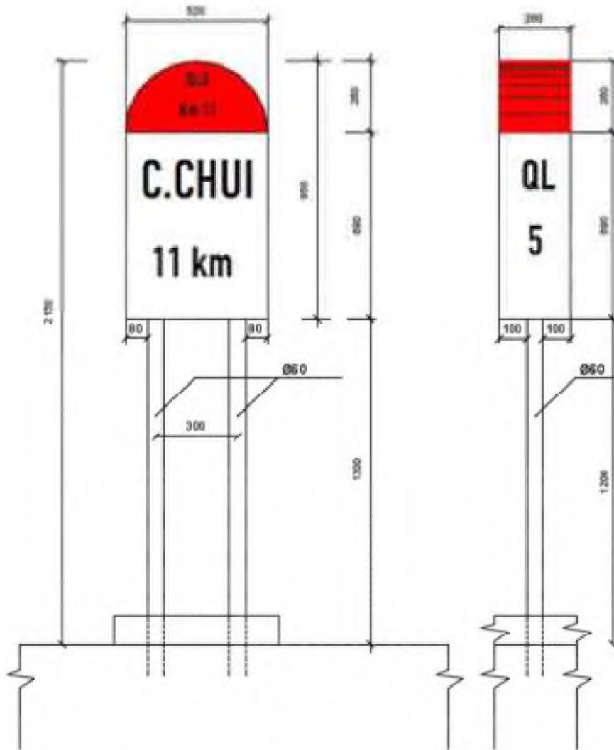
Ghi chú: Kích thước ghi trên hình vẽ là mm Hình I.2 - Cột kilômét dạng cột cao
