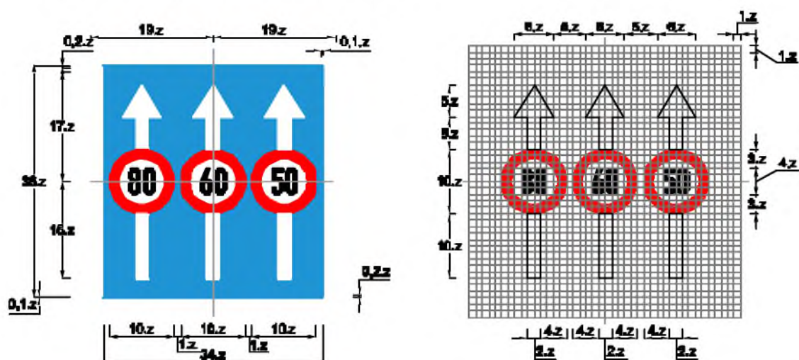
Biển số P.127b: Biển gộp tốc độ tối đa cho phép theo làn đường đặt bên đường hoặc trên cột đèn vôn
