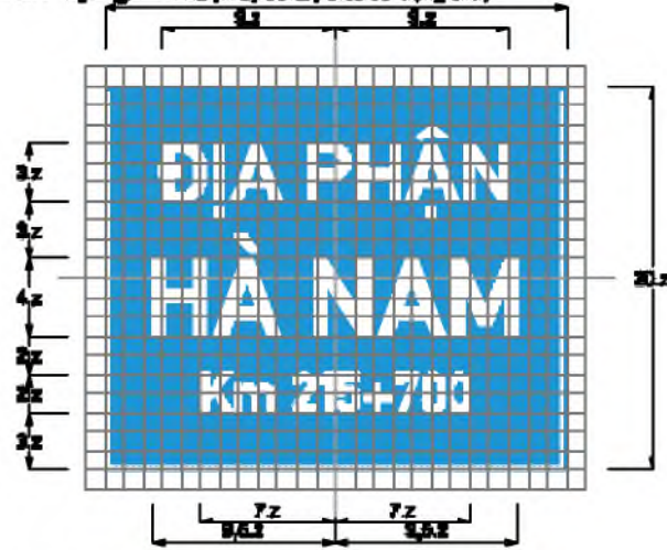
Biển 419b : Chỉ dẫn địa giới trên tuyến đường đối ngoại
