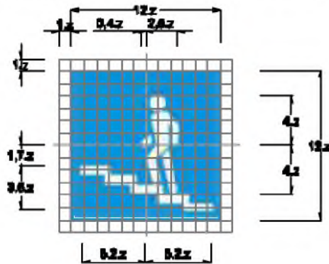
Biển số I.424b : Cầu vượt qua đường cho người đi bộ
