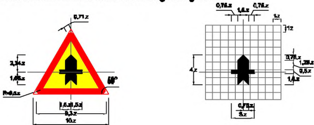
Biển số W.207a: Giao nhau với đường không ưu tiên
