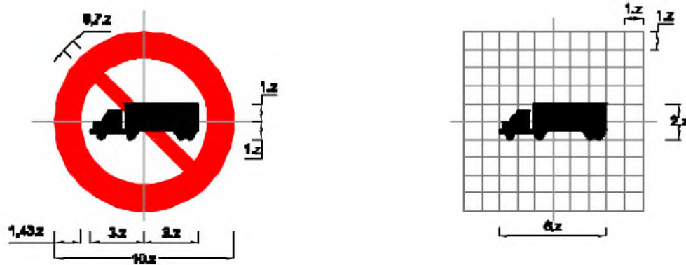
Biển số P.108a: Cấm xe sơ-mi-ro-môóc
