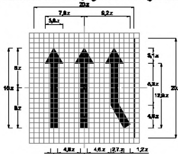
Biển số S.G.11c: Biển chỉ dẫn số lượng làn và hướng đi cho từng làn
