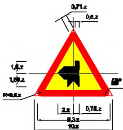
Biển số W.207k: Giao nhau với đường không ưu tiên
