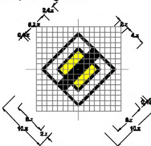
Biển số I.402: Hết đoạn đường ưu tiên
