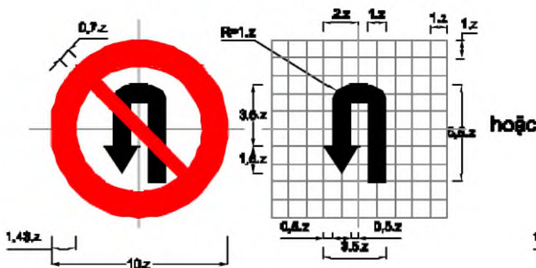
Biển số P.124a: Cấm quay đầu xe
