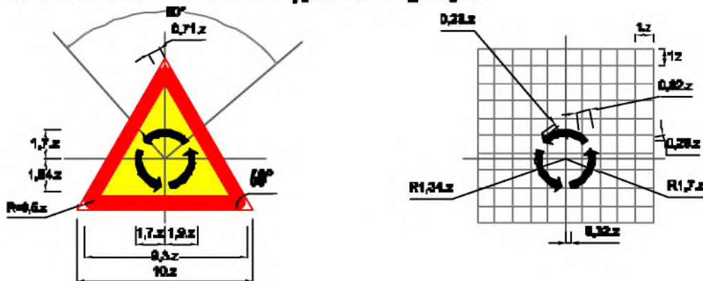
Biển số W.206: Giao nhau chạy theo vòng xuyến
