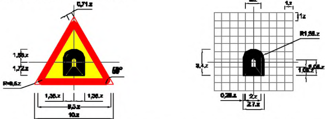
Biển số W.240: Đường hầm
