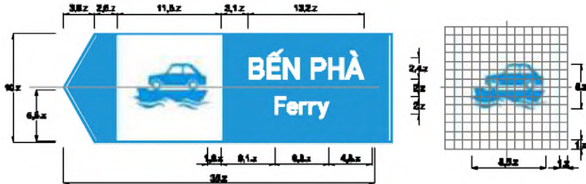
Biển số 1.444j : Biển báo chỉ dẫn địa điểm
